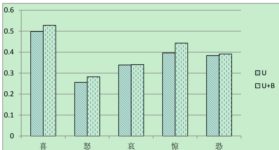
图 3: 使用 Unigram 和 Unigram+Bigram 特征得到的分类结果比较
