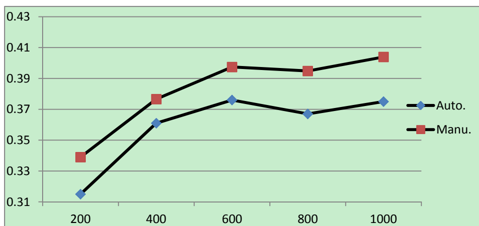
图 4: 使用不同训练样本规模的情绪分类结果
