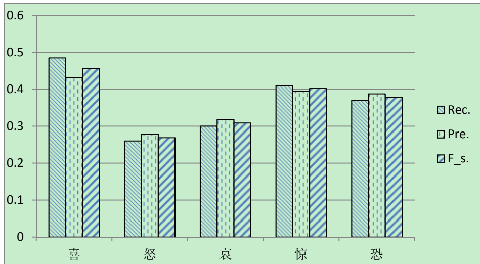
图 1: 上下文方法在自动标注测试语料上面的情绪分类结果
