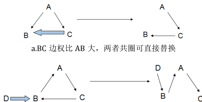
a. BC 边权比 AB 大，两者共圈可直接替换 b. ABC 是替换后产生的环，DB 是符合要求的未选边，损失最小的边权来打开环 图 2 最小树形图算法思路图解
