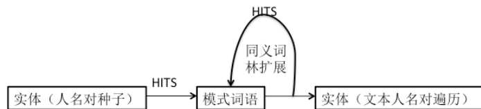
图 1. 改进后的实体和模式提取流程
