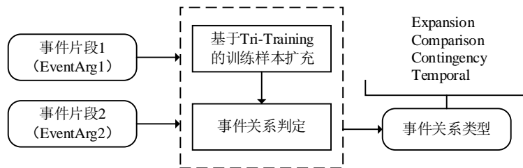
图3 事件关系分类任务框架
