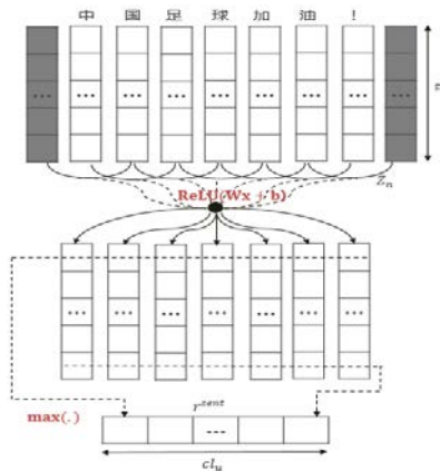
图 1 基于卷积方法抽取句子级别特征
