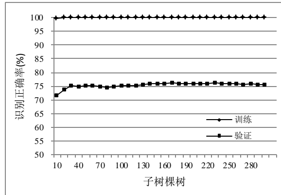
图 4 不同子树数量的随机森林训练和验证结果
