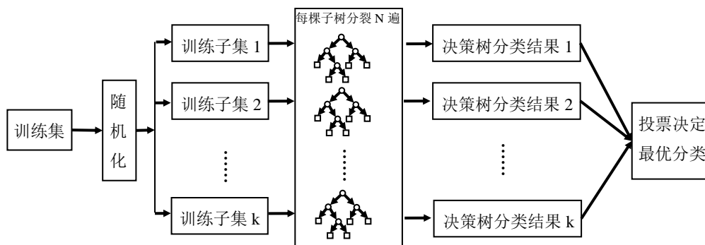
图 3 随机森林训练原理示意图
