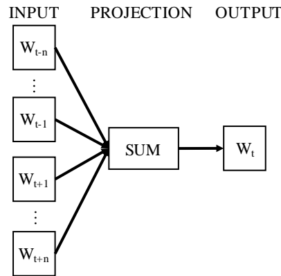
图 2 CBOW 语言模型架构
