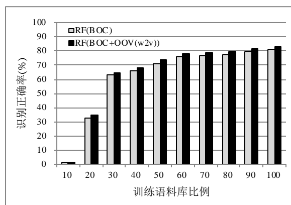
图 7 不同比例训练语料的测试结果
