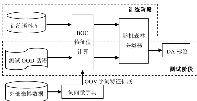
图 1 限定领域口语对话系统 OOD 话语 DA 识别方法技术架构
