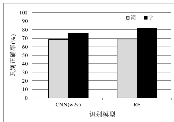
图 5 不同原始特征（词和子）的 DA 识别效果
