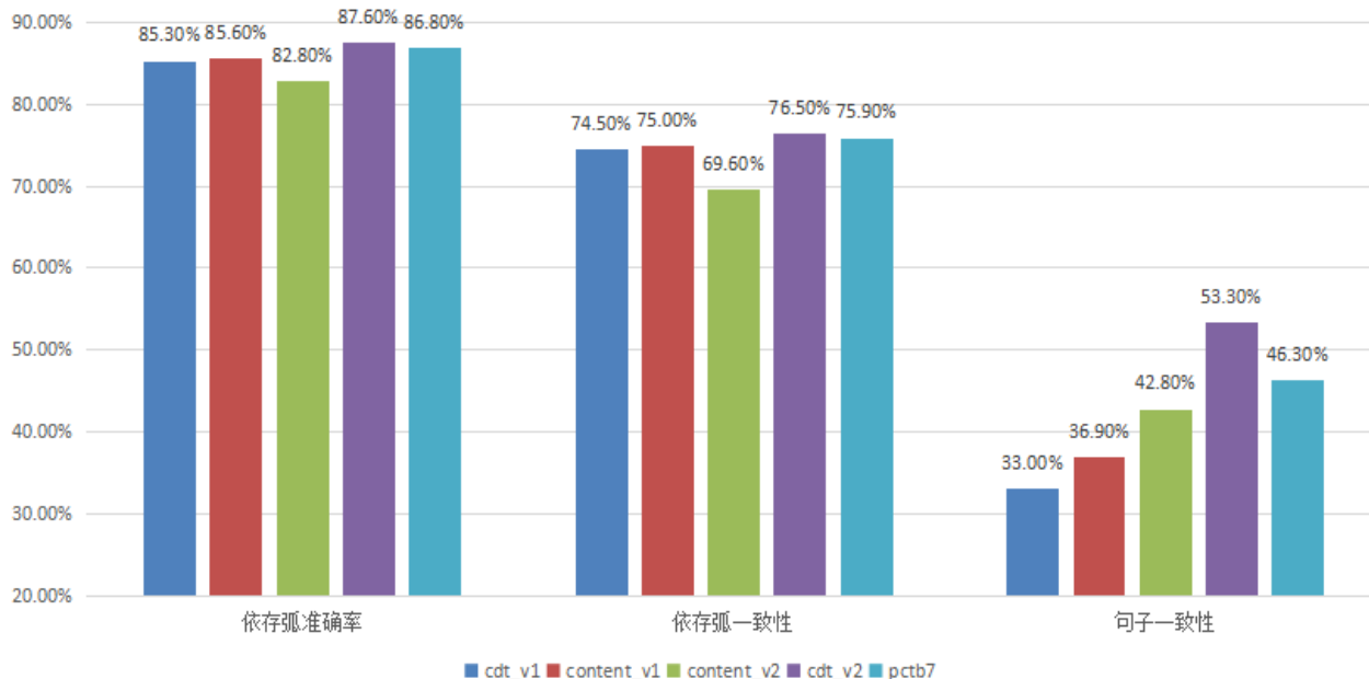
图 3 各批次整体评价指标
