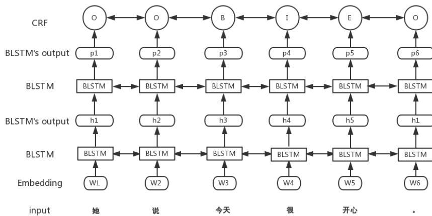
图 1 引语识别的 BLSTM-CRF 模型
