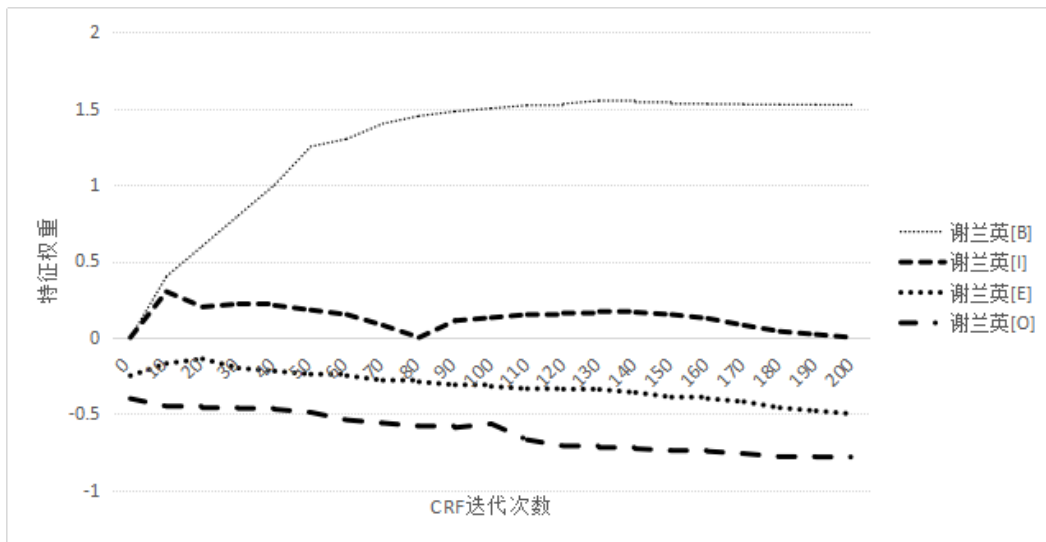
图 3 引入管领词特征“谢兰英”特征权重变化图
