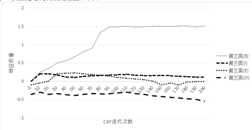
图 4 不引入管领词特征“谢兰英”特征权重变化图
