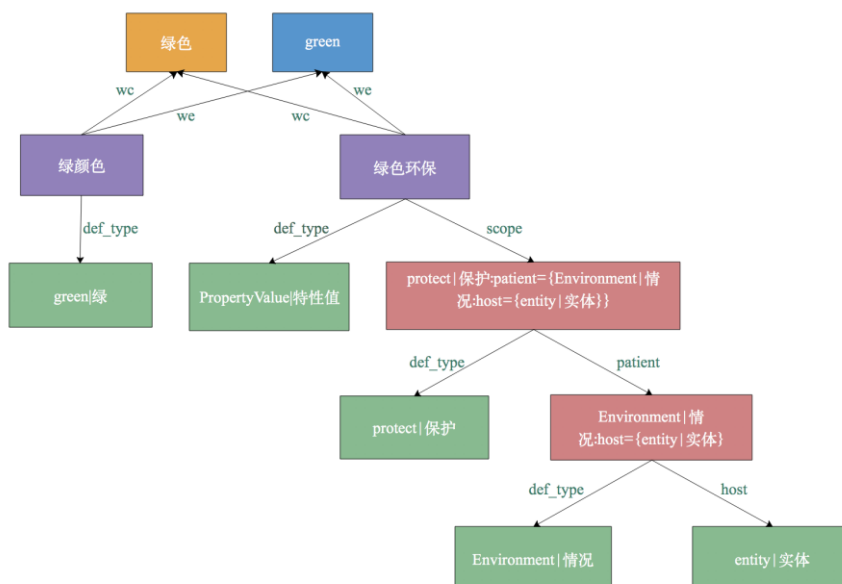
图3 HownetGraph 中“绿色”的子图表示。方框表示实例，颜色表示所属的概念：黄色表示中文词语，蓝色表示英文词语，紫色表示义项，绿色表示义原，红色表示 DEF_CONCEPT。边表示关系：wc 表示义项的中文词，we 表示义项的英文词，def_type 表示义项或 DEF_CONCEPT 的基本义原，scope、patient 和 host 分别表示义项或 DEF_CONCEPT 的范围、受事和宿主关系。
