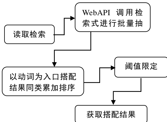
图 8 介词结构搭配抽取流程图
